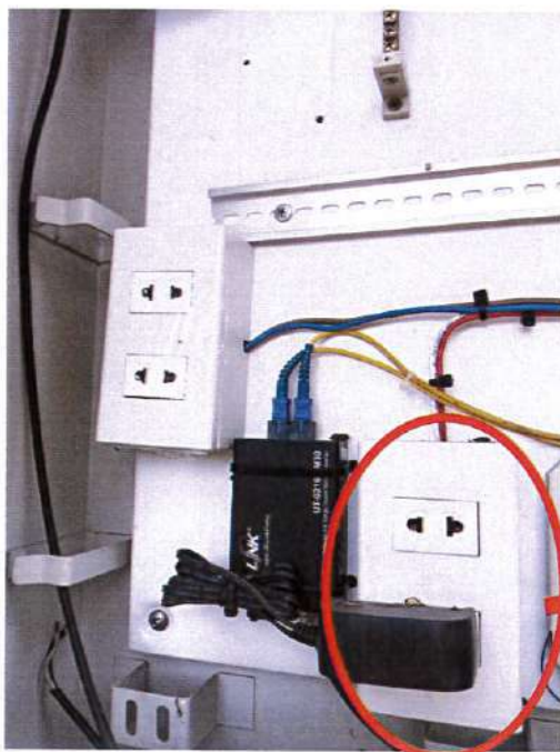
รูปภาพ ชุดบล็อกปลั๊กไฟ ๒๒๐V อันเดิม ช่องเสียบแตกข้างใน ต้องเปลี่ยน
