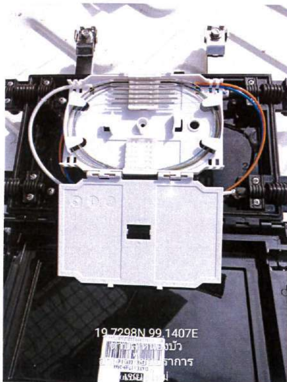
รูปภาพการต่อเคเบิลในอุปกรณ์ Closure Splice Snap Lock (หัว ๑ กล่อง -ท้าย ๑ กล่อง)
