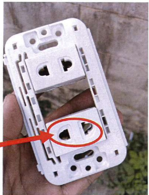
รูปภาพ ชุดบล็อกปลั๊กไฟ ๒๒๐V อันเดิม ช่องเสียบแตกข้างใน ต้องเปลี่ยน
