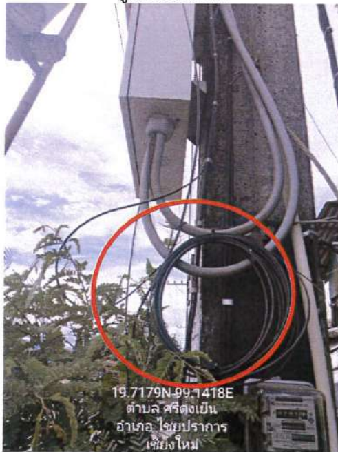
รูปภาพ การตัดต่อหัว-ท้าย ของสายสัญญาณ Fiber Optic ๑ core
