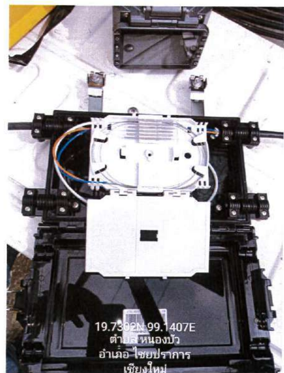
รูปภาพการต่อเคเบิลในอุปกรณ์ Closure Splice Snap Lock (หัว ๑ กล่อง -ท้าย ๑ กล่อง)
