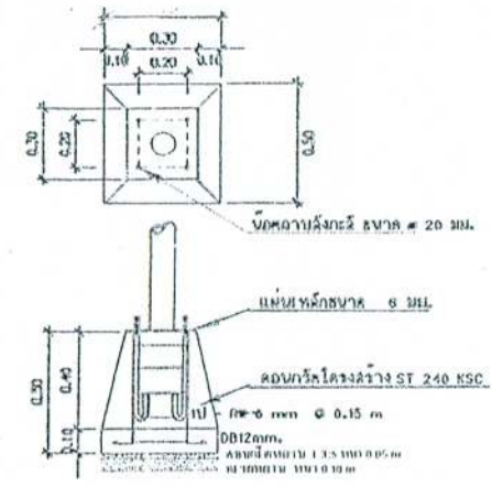
แบบขยายฐานราก มาตราส่วน 1:34
