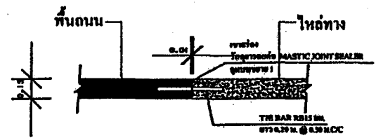
ขยายรอยต่อ LONGITUDINAL JOINT NOT TO SCALE
