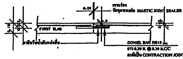
ขยายรอยต่อ CONTRACTION JOINT ทุกระยะ 4.00 ม. NOT TO SCALE
