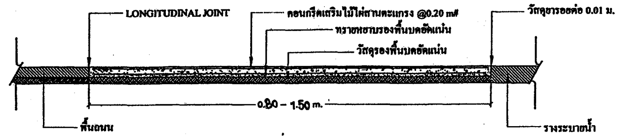
รูปตัด โครงสร้างพื้น คตม. ขนาด 1:20
